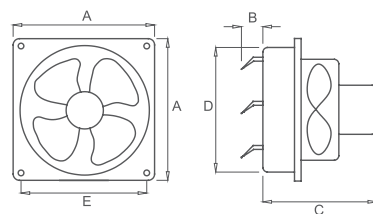
EXTRACTOR TRITÓN
